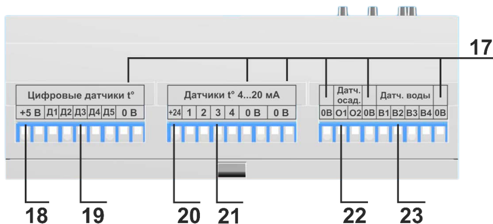
Рисунок 3. Вид снизу
