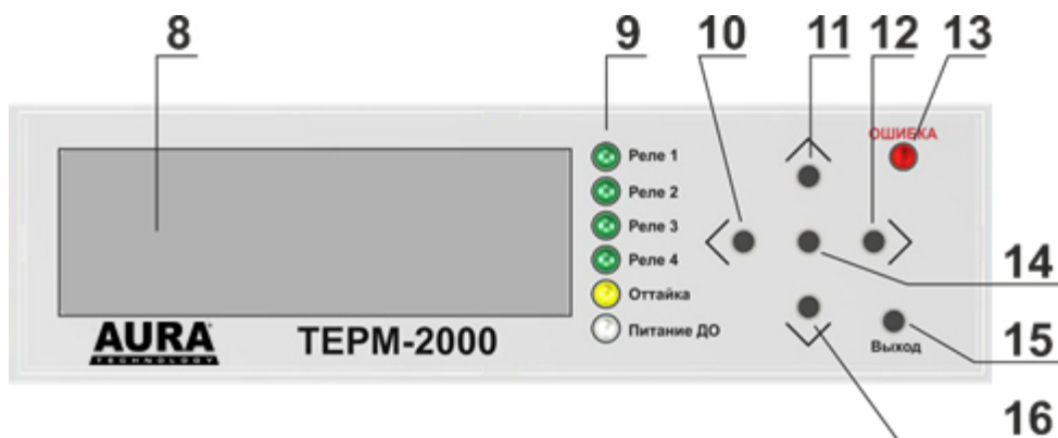
Рисунок 2. Лицевая панель
